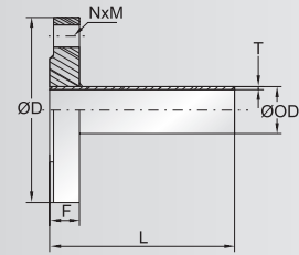
Pipe flange
